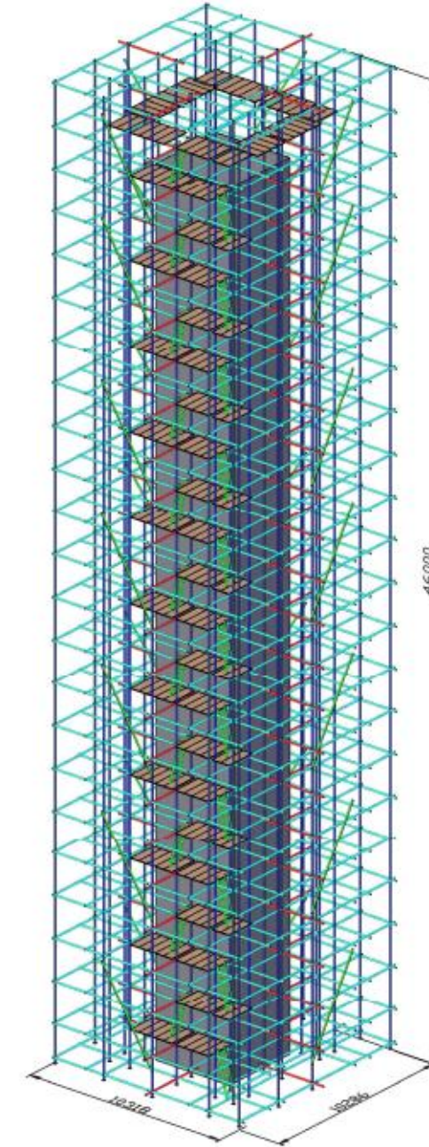
Изометрический вид
