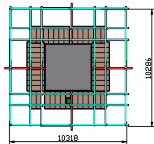
Вид сверху
