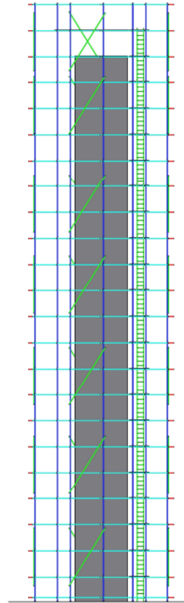
Вид сбоку
