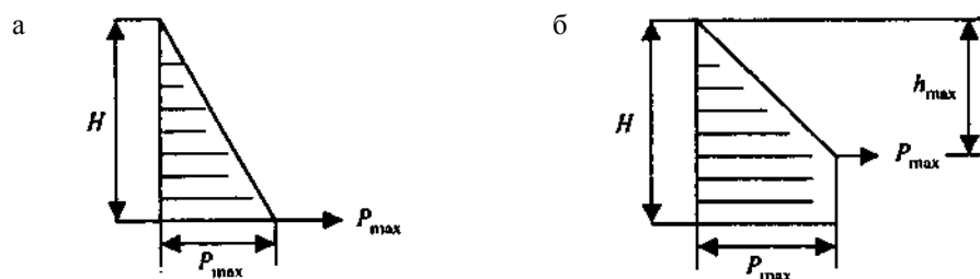
Рисунок Г.1 — Расчетные эпюры бокового давления бетонной смеси а — гидростатическое давление; б — расчетное давление при уплотнении смеси внутренними вибраторами
